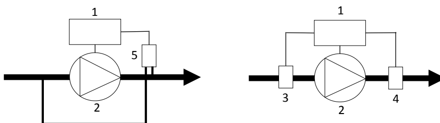
1: Wechselrichter; 2: Pumpe; 3: Drucksensor; 4: Drucksensor; 5: Differenzdrucksensor
