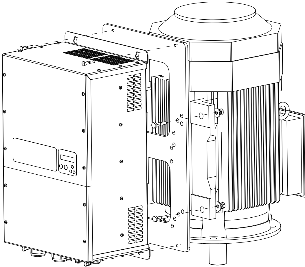
Abbildung 1. Motorkit für Geräte der Größe 3
